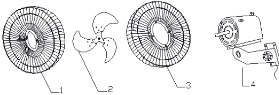
1) ÖN KAFES 2) PERVANE 3) ARKA KAFES 4) MOTOR ve DUVAR APARATI
